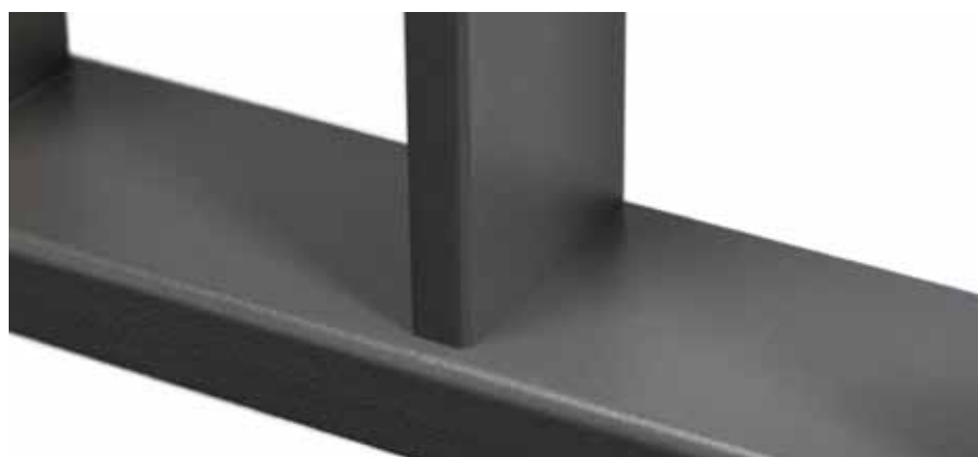
Geen lasverbinding meer noodzakelijk bij de aansluiting van kokers
