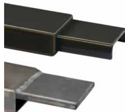
Geen lasverbinding meer noodzakelijk bij de aansluiting van kokers
